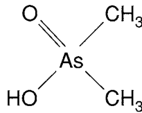
Fig. 15. Cacodylic acid.
